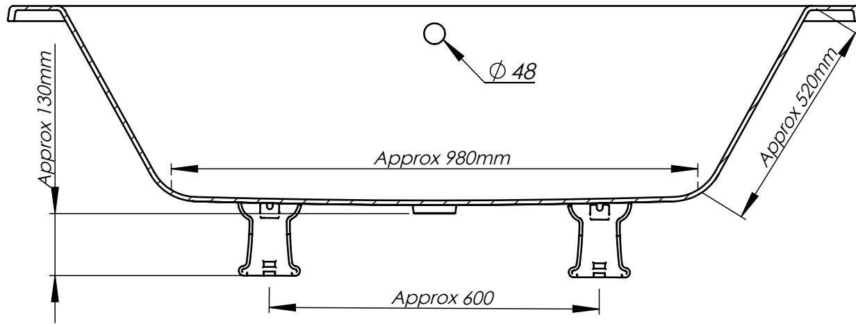
PROFILE A-A
